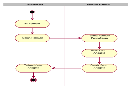
Gambar 1. Activity Diagram Pendataan Data anggota
