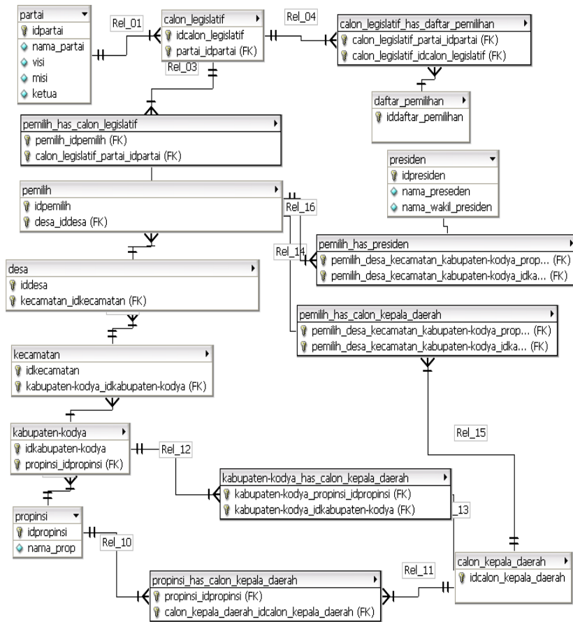
Gambar 6 Hubungan antar tabel untuk sistem yang diusulkan
