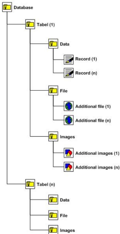
Gambar 1 Struktur Direktori
