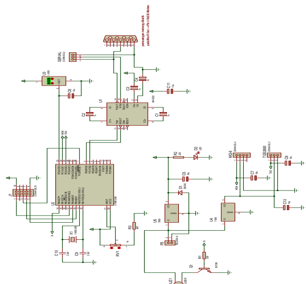
Gambar 3. Skema Rangkaian
