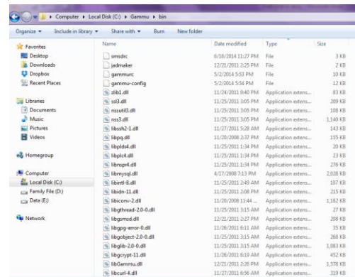
Gambar 4.1 Implementasi Gammu
