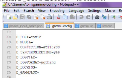
Gambar 4.4 Konfigurasi Gammu-Config
